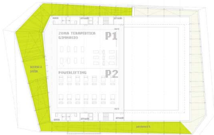
planta entreplanta (cota +4.00) e 1/400
