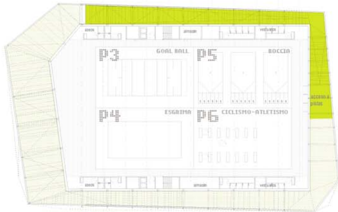
planta primera (cota +9.50) e 1/400
